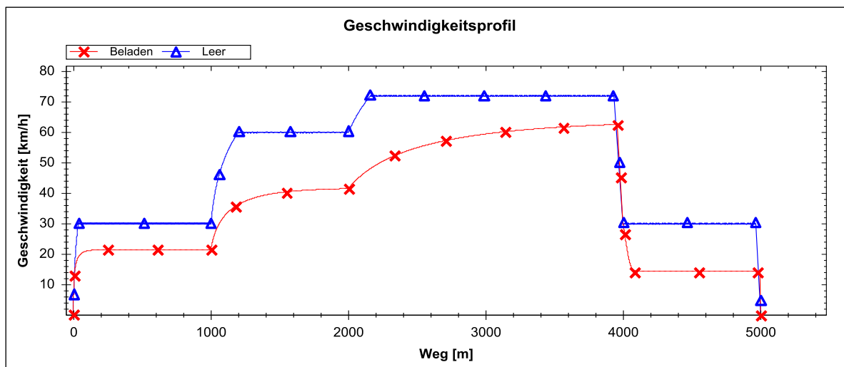
Abbildung 3: Simuliertes Geschwindigkeitsprofil
