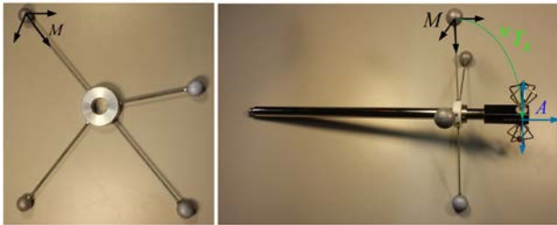
Abbildung 8. Marker einzeln (links) und Antenne mit Marker zur Messung (rechts) der Pose der Feldstärkemessung
